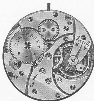
18''' Lép. Sav. 590 591 592 593 40,25 mm. H. 4,30 mm.
