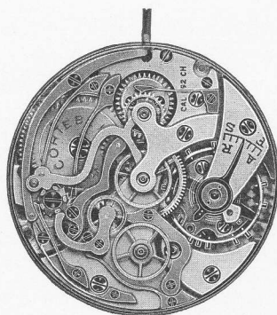
18''' - 582 Chronogr. 40,25 mm. H. 6,00 mm.
