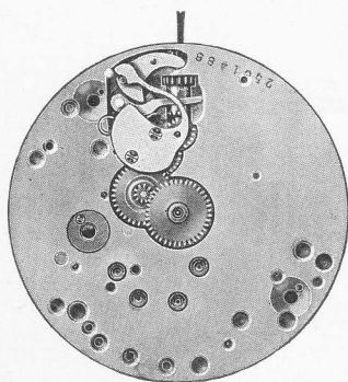
18''' - 582 Chronogr. 40,25 mm. H. 6,00 mm.
